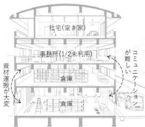
改修前南北断面パース
